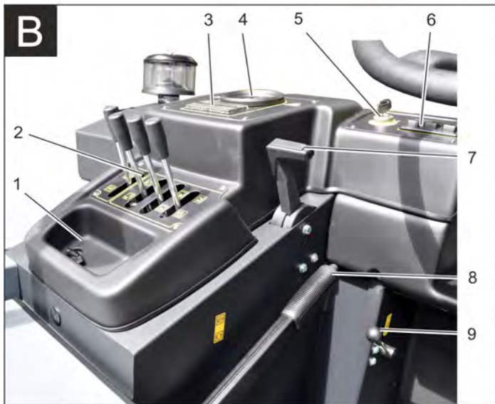
Εικόνα μηχανικού σαρώθρου
