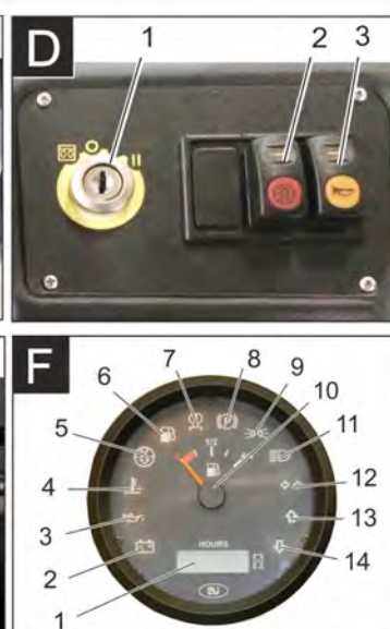
Kontaktna brava / funkcijski tastere
